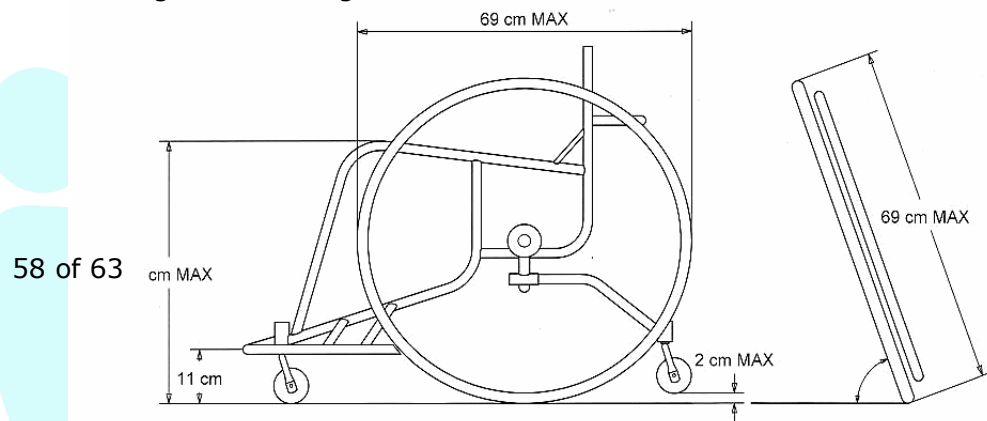
Figuur : afmetingen van de basketbalrolstoel
